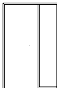
Zarge mit Kämpfer für Drehtür mit Seitenteil
